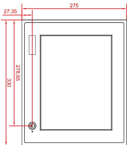
CP6901-0010 main dimensions
