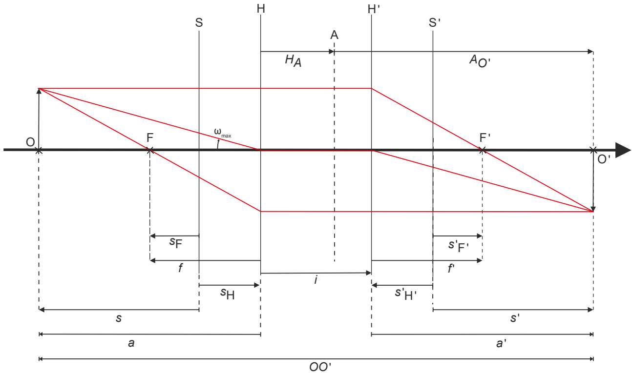
Abb. 4: Geometrische Optik
