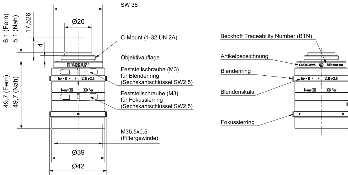
Abb. 3: Technische Zeichnung
