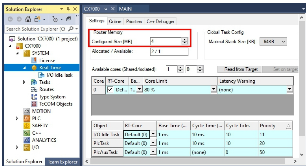
Abb. 68: Einstellungen für Router-Speicher im TwinCAT System Manager.
