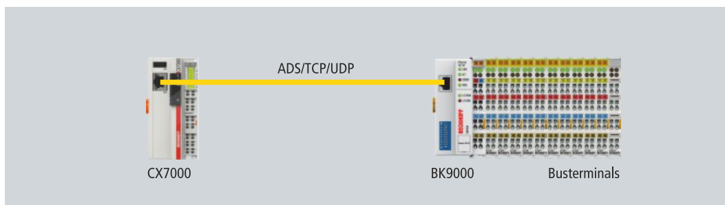
Abb. 45: Virtuelle Ethernet-Kommunikation über ADS, TCP oder UDP.
