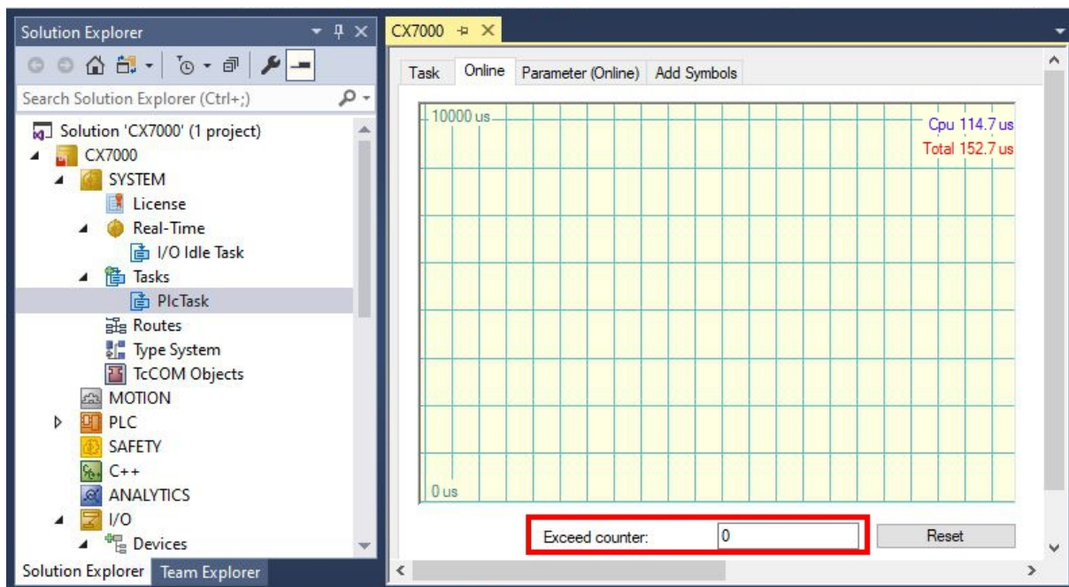
Abb. 70: Anzeige des Exceed-Counters in TwinCAT.
