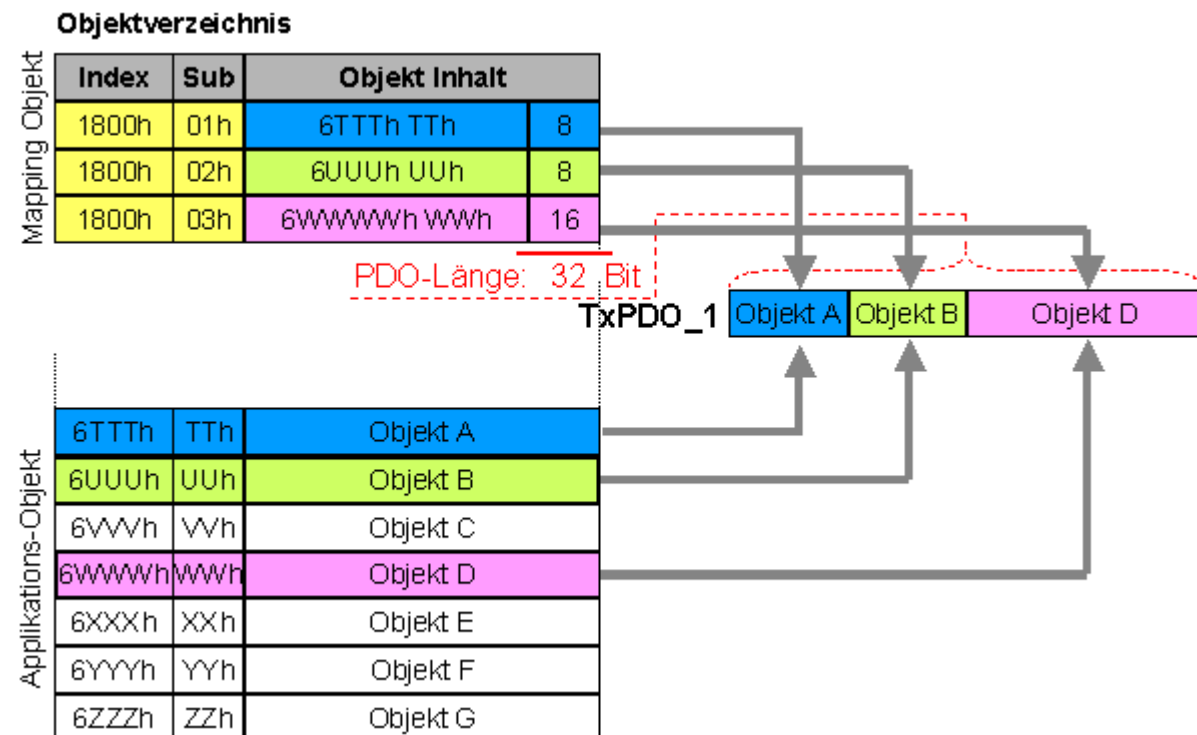
Abb. 15: Darstellung Mapping
