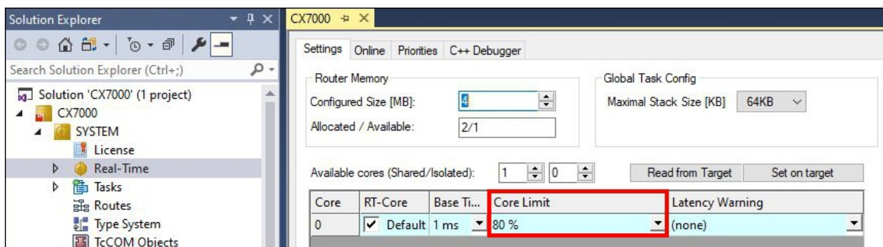
Abb. 72: Einstellung der Echtzeitauslastung in TwinCAT.
