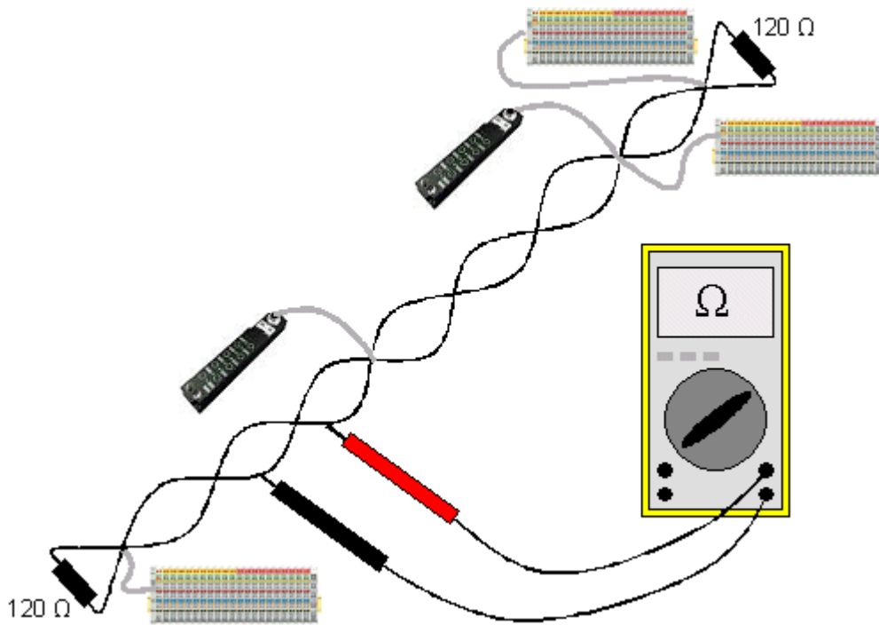
Abb. 65: Verdrahtungsplan für Testaufbau
