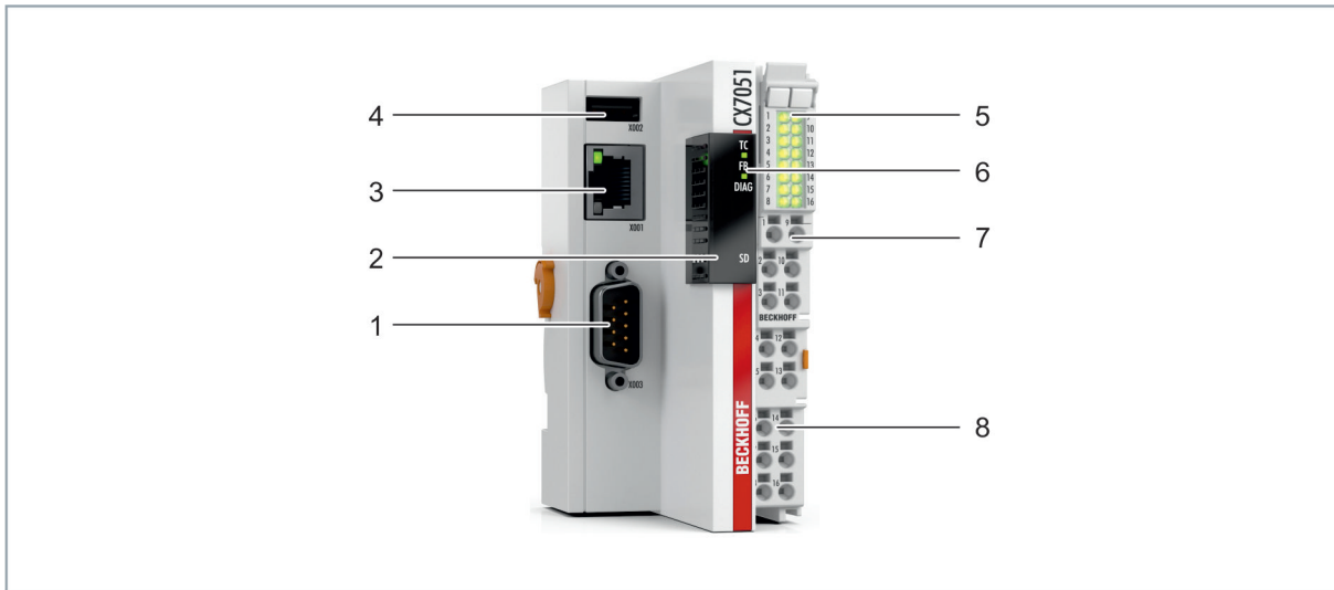
Abb. 1: Beispielaufbau eines Embedded-PCs CX7051.
