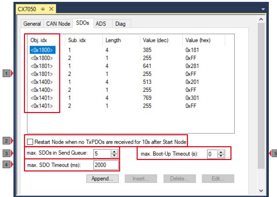
Abb. 41: SDO-Registerkarte eines CANopen-Slaves in TwinCAT.
