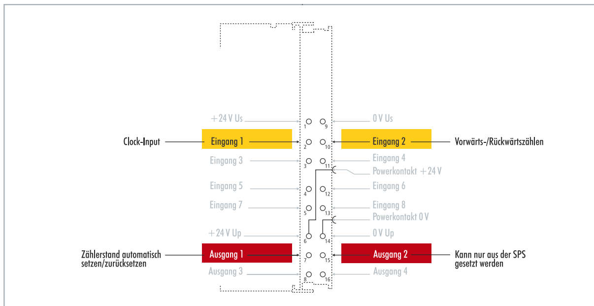
Abb. 32: Konfigurierbare Ein- und Ausgänge im Zähler-Modus.
