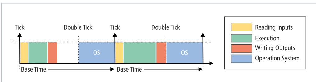
Abb. 55: Standard-Aufruf einer SPS-Task.
