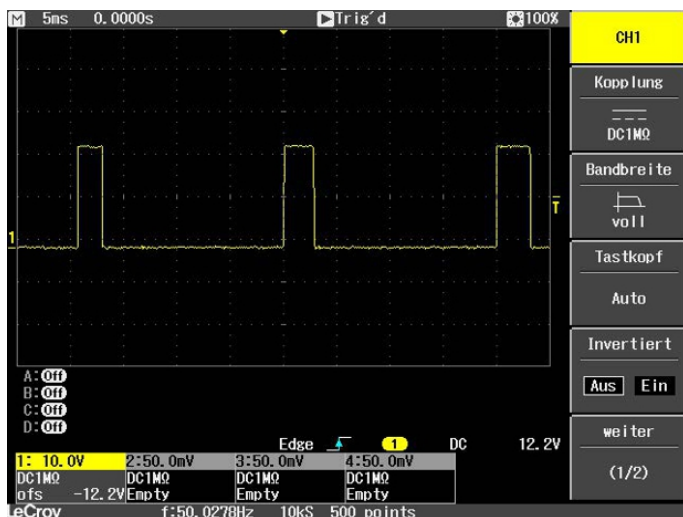
Abb. 58: Verkürzter Puls eines digitalen Ausgangs mit Last.
