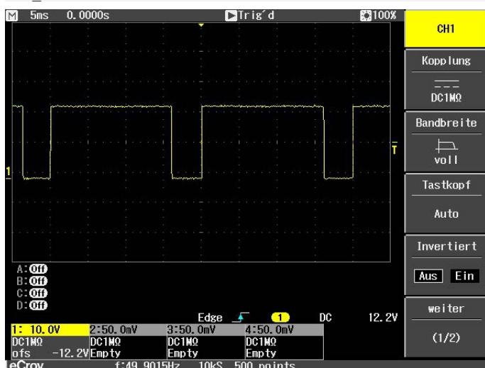
Abb. 59: Invertierte Darstellung eines digitalen Ausgangs.
