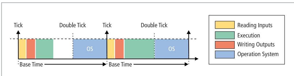
Abb. 56: Aufruf einer SPS-Task mit Attribut TcCallAfterOutputUpdate.
