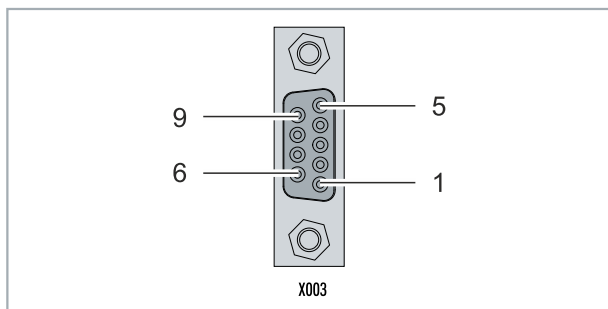
Abb. 4: PROFIBUS-Schnittstelle X003.
