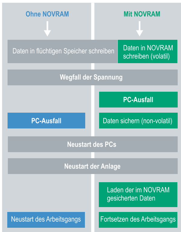
Abb. 24: Verhalten der Steuerung ohne und mit NOVRAM.
