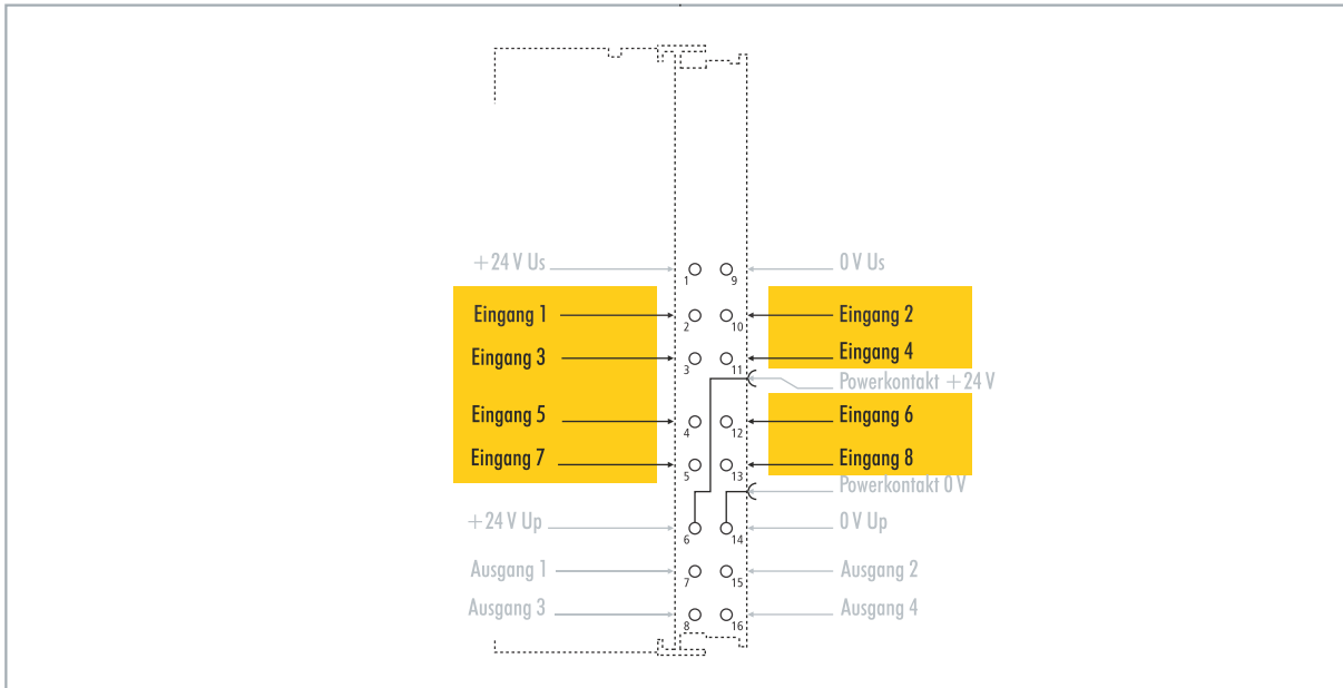
Abb. 18: Konfigurierbare digitale Eingänge.
