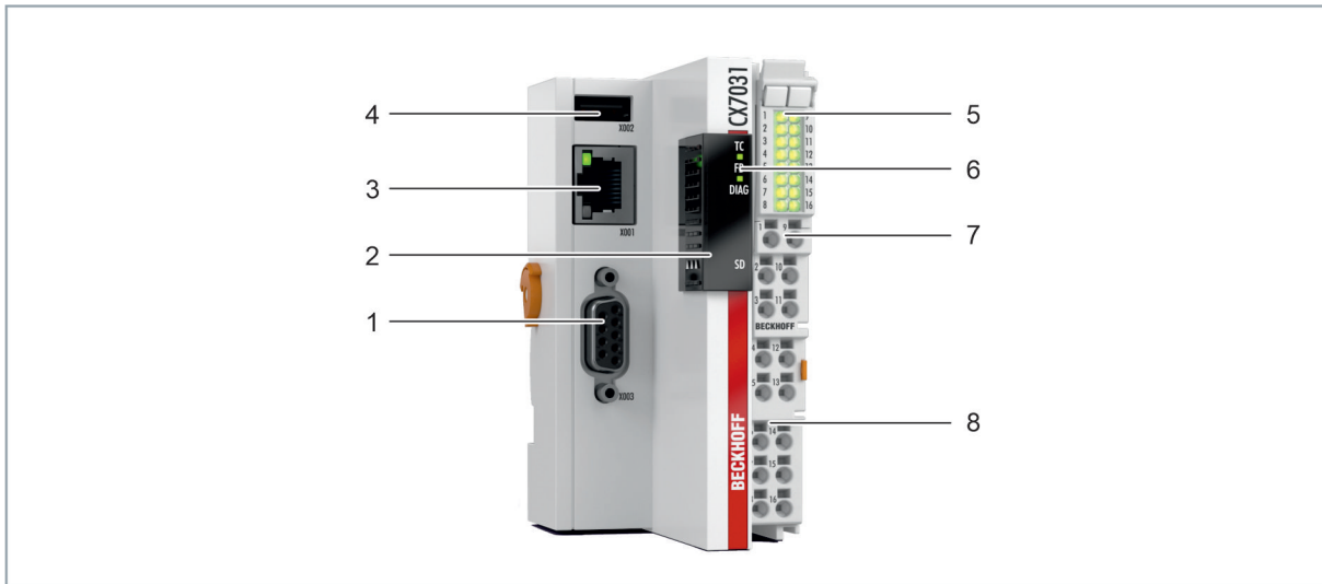
Abb. 1: Beispielaufbau eines Embedded-PCs CX7031.
