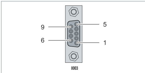
Abb. 12: PROFIBUS-Schnittstelle X003.
