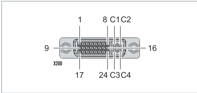
Abb. 7: DVI-I-Schnittstelle X200.
