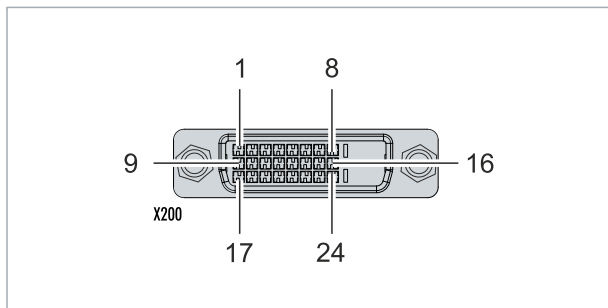
Abb. 8: DVI-D-Schnittstelle X300.
