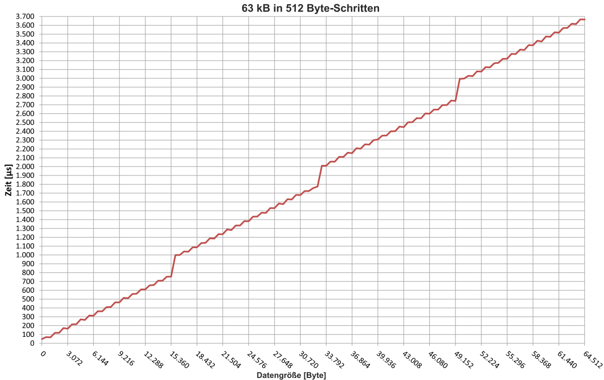
Abb. 35: Retain-Handler Schreibgeschwindigkeit, bis 63 kB in 512 Byte-Schritten.
