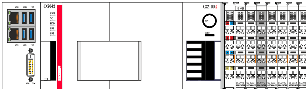
Abb. 24: Passive EtherCAT-Klemmen, zulässige Montage.
