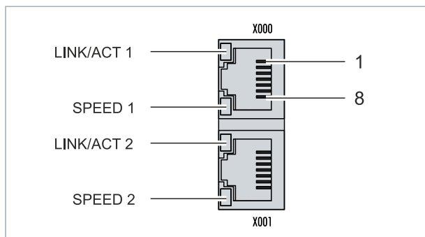
Abb. 6: Ethernet-Schnittstellen X000, X001.
