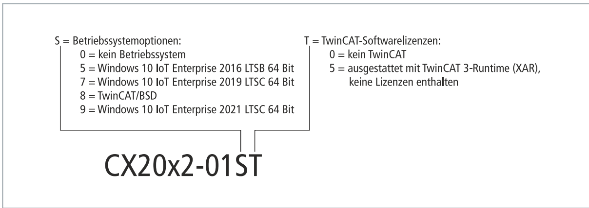
Abb. 3: Bezeichnungssystematik des CPU-Grundmoduls.
