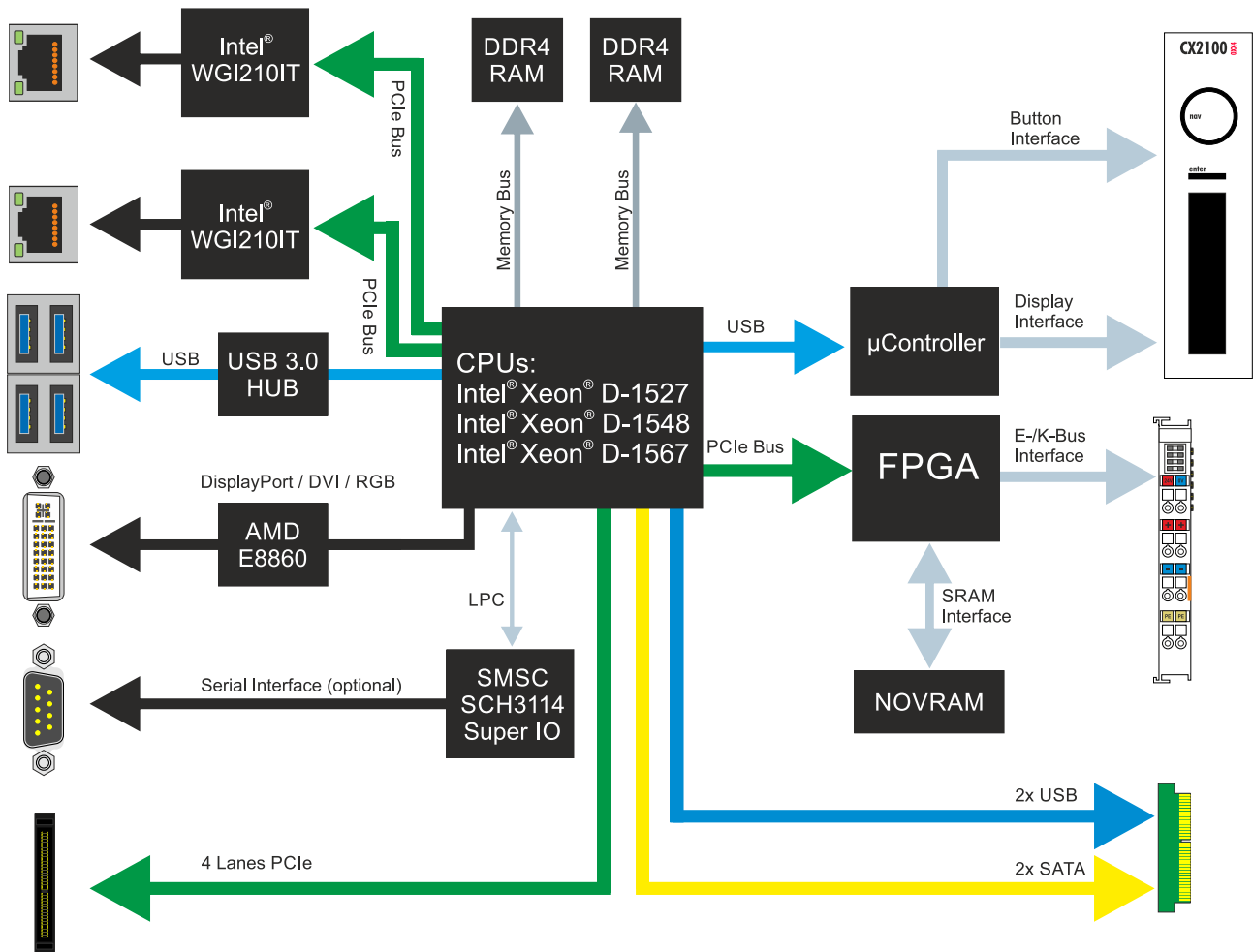
Abb. 4: CX20x2 Architekturübersicht.
