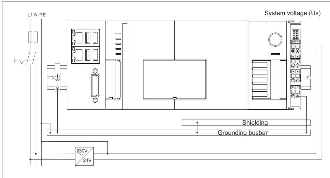
Abb. 27: Anschlussbeispiel mit einem CX20x2.
