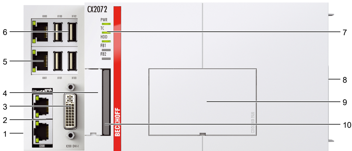
Abb. 1: Beispielaufbau eines Embedded-PCs CX2072.
