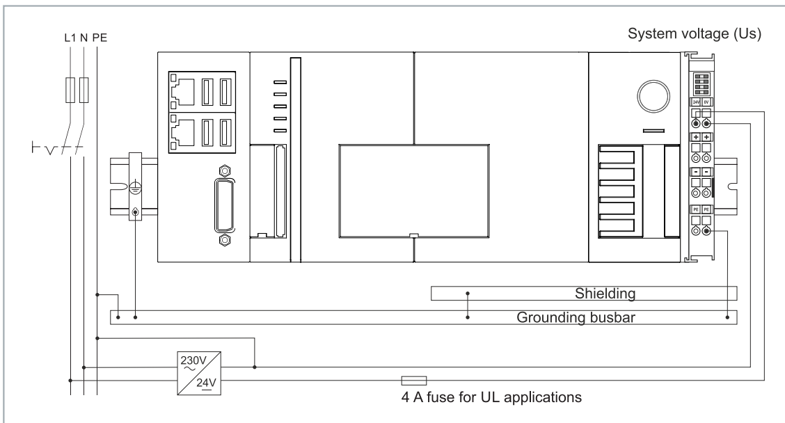
Abb. 29: Anschlussbeispiel für Bereiche mit speziellen UL-Anforderungen.
