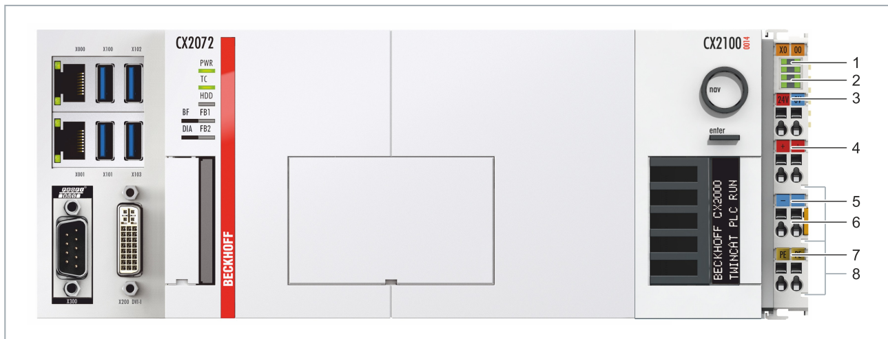
Abb. 19: Embedded-PC CX20x2 mit Netzteil CX2100-0014, Aufbau der Netzteilklemme.
