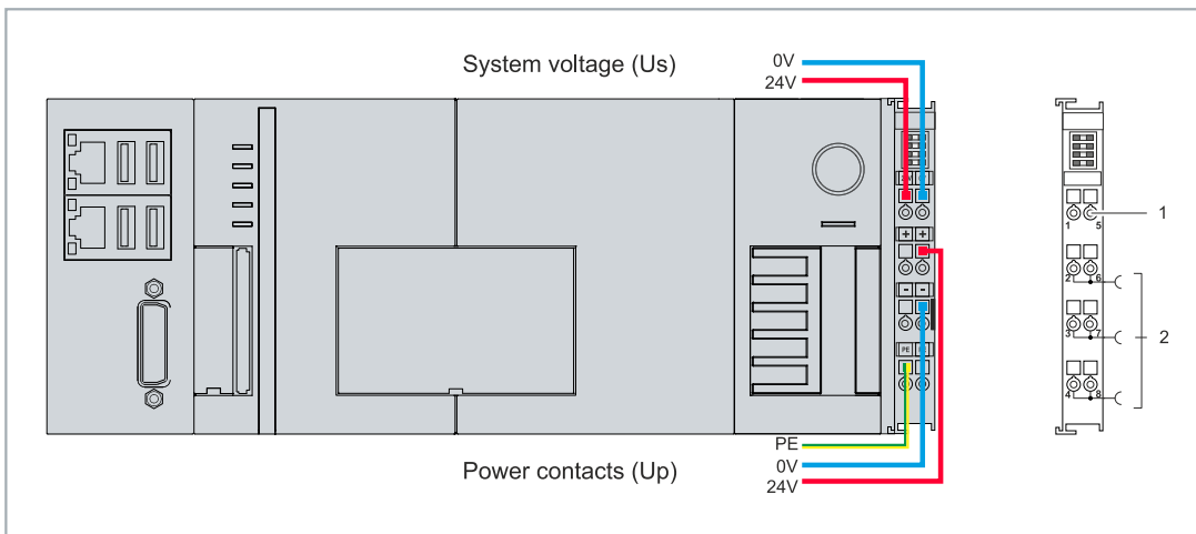
Abb. 26: Anschlüsse für Systemspannung (Us) und Powerkontakte (Up).
