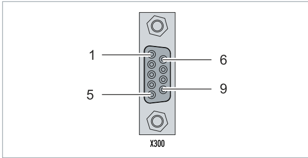
Abb. 13: RS485-Schnittstelle X300.
