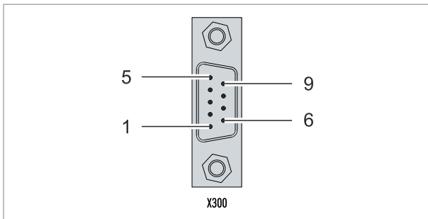
Abb. 12: RS232-Schnittstelle X300.
