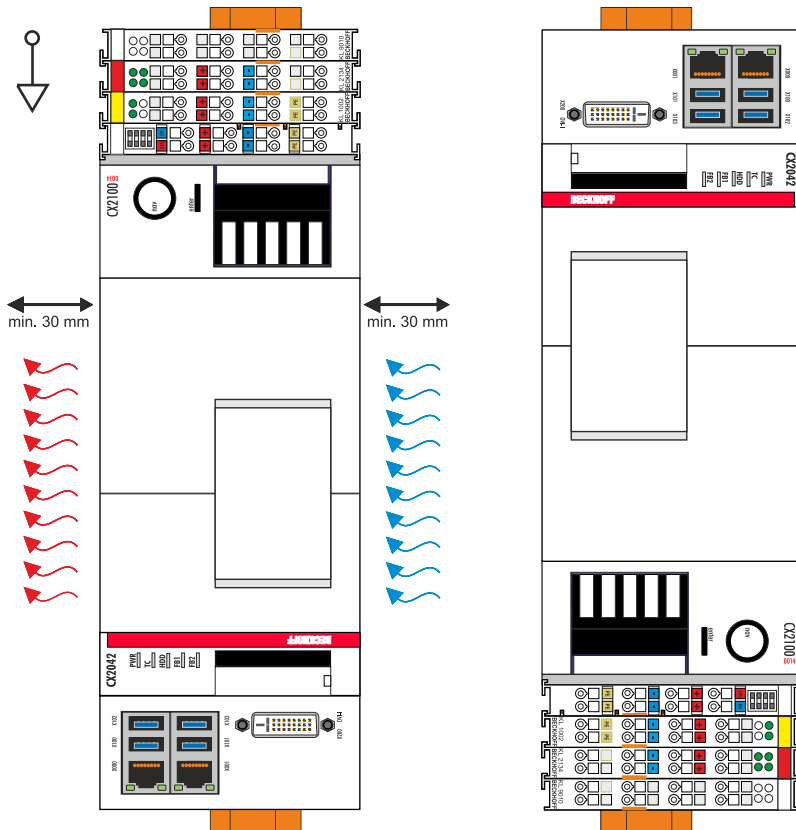
Abb. 21: Embedded-PC CX20x2, senkrechte Einbaulage.
