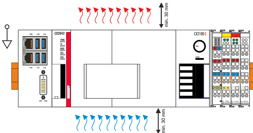
Abb. 20: Embedded-PC CX20x2, waagrechte Einbaulage.
