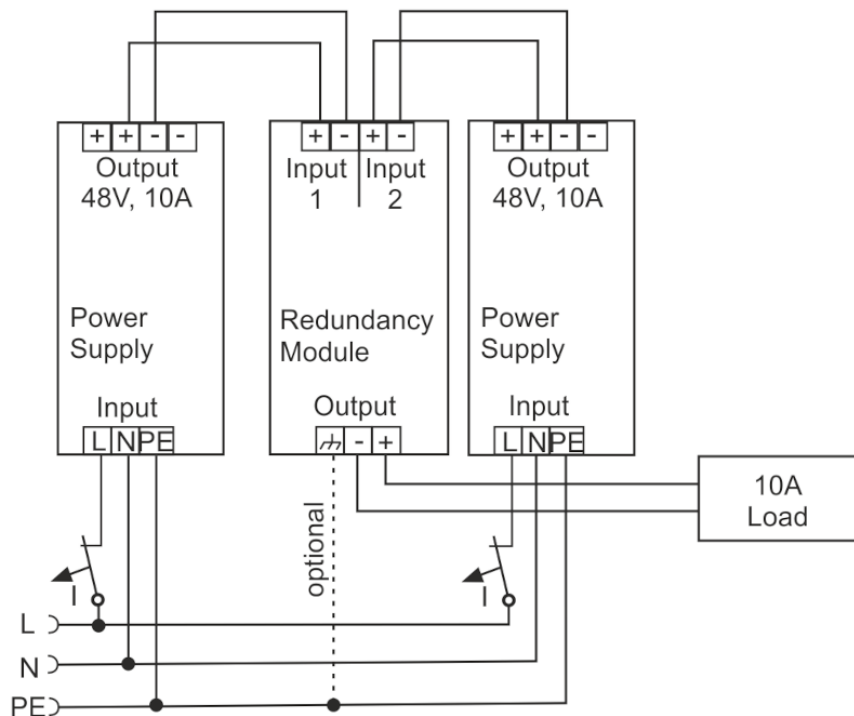
Abb. 23: Verdrahtung für 1+1 - Redundanz mit einem Redundanzmodul PS9421-4840-0000
