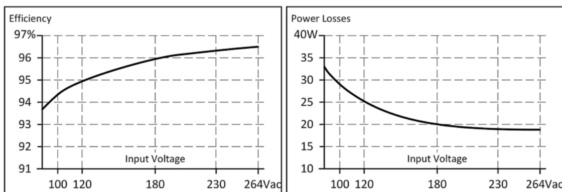
Abb. 10: Wirkungsgrad zu Eingangsspannung bei 48V, 10 A, typ.; Verluste zu Eingangsspannung bei 48V, 10 A, typ
