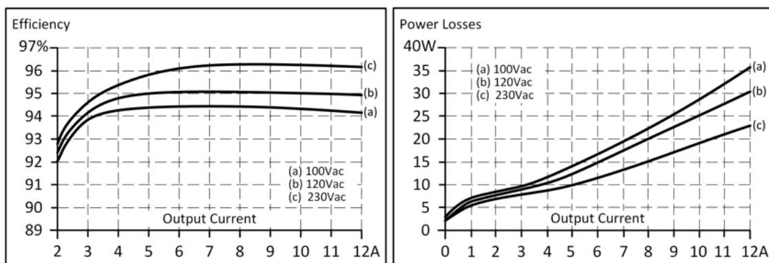
Abb. 9: Wirkungsgrad zu Ausgangsstrom bei 48 V typ.; Verluste zu Ausgangsstrom 48 V typ.
