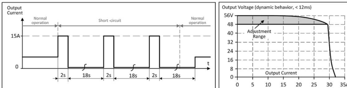
Abb. 7: Kurzschluss am Ausgang, Hiccup-Modus, typ.
