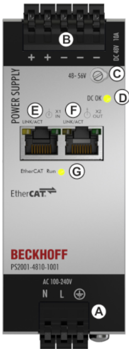
Abb. 13: Vorderseite PS2001-4810-1001
