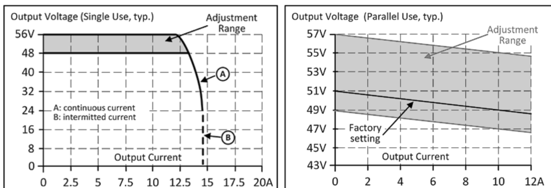
Abb. 6: Ausgangsspannung zu Ausgangsstrom (single use); Ausgangsspannung zu Ausgangsstrom (parallel use)
