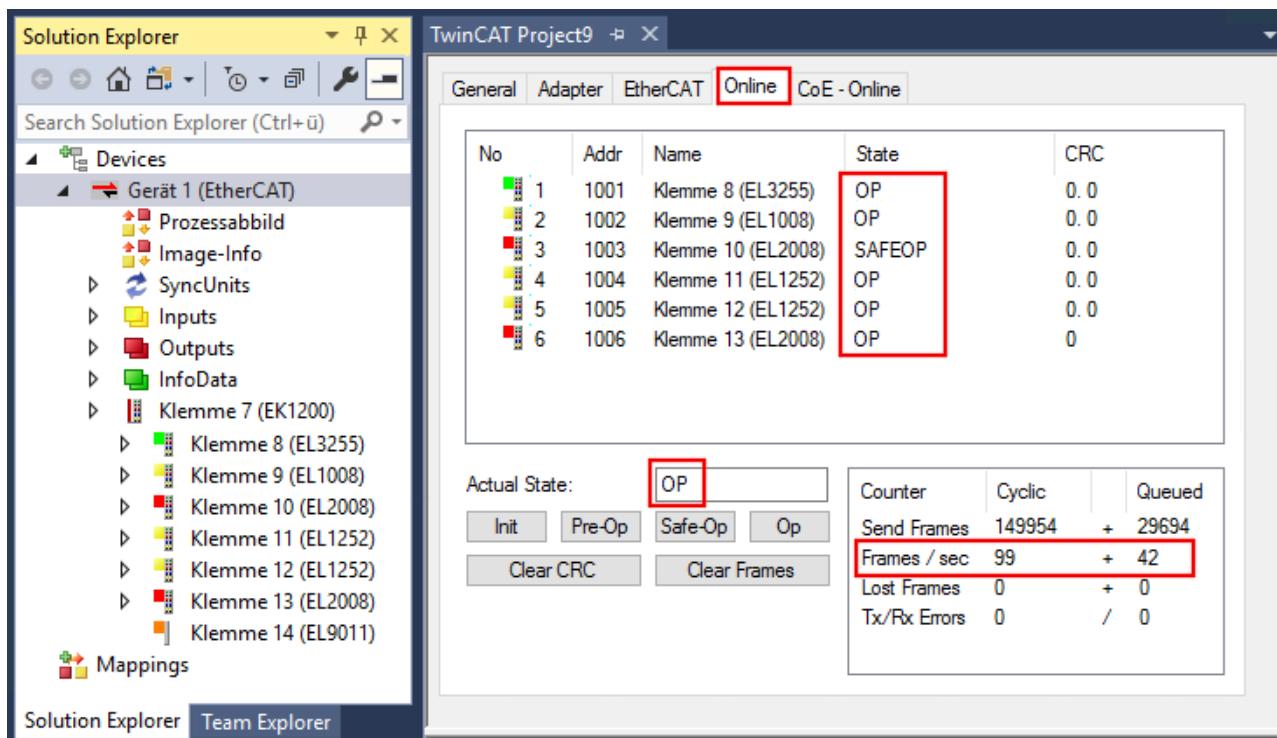
Abb. 93: Beispielhafte Online-Anzeige
