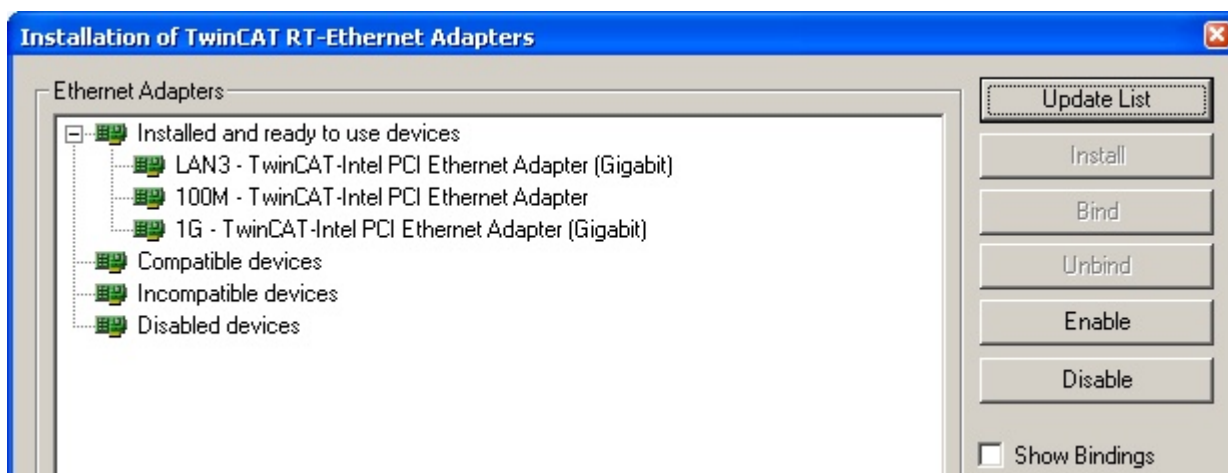
Abb. 59: Übersicht Netzwerkschnittstellen
