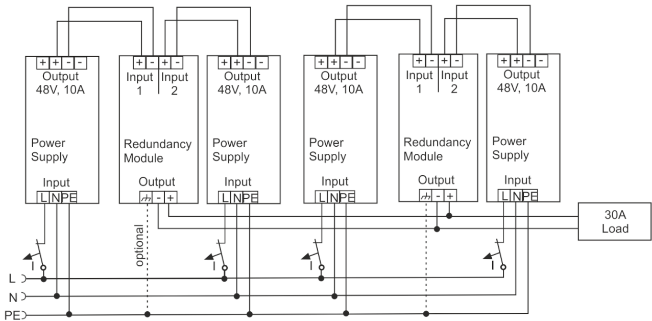
Abb. 24: Verdrahtung für n+1 - Redundanz mit zwei Redundanzmodulen PS9421-4840-0000
