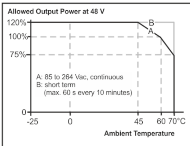
Abb. 14: Ausgangsleistung zu Umgebungstemperatur; Ausgangsleistung zu Aufstellhöhe
