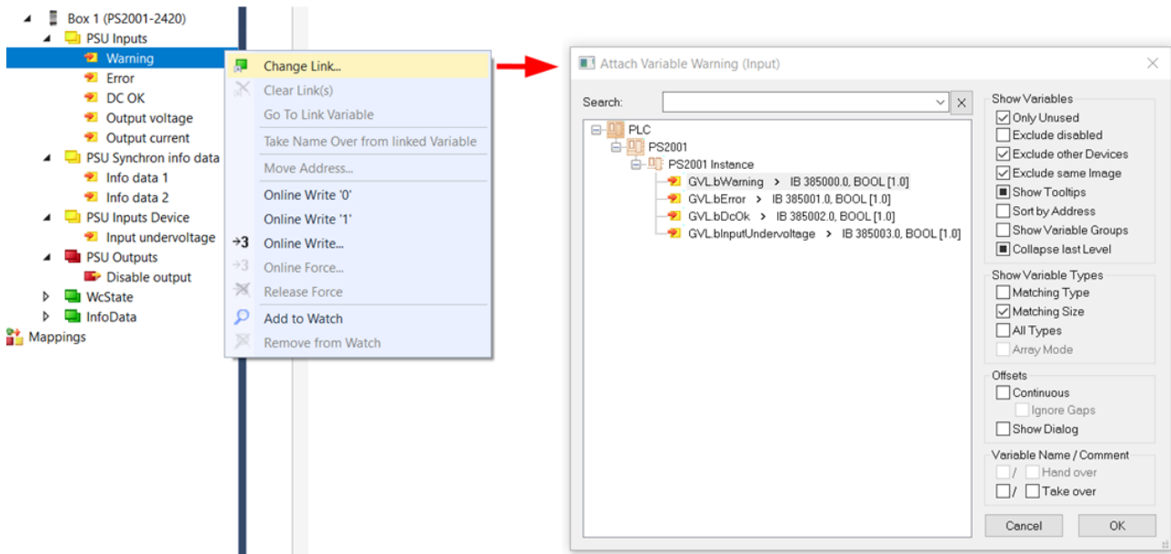
Abb. 119: Verknüpfung des Warning-Bits aus den Prozessdaten mit der PLC-Variable bWarning
