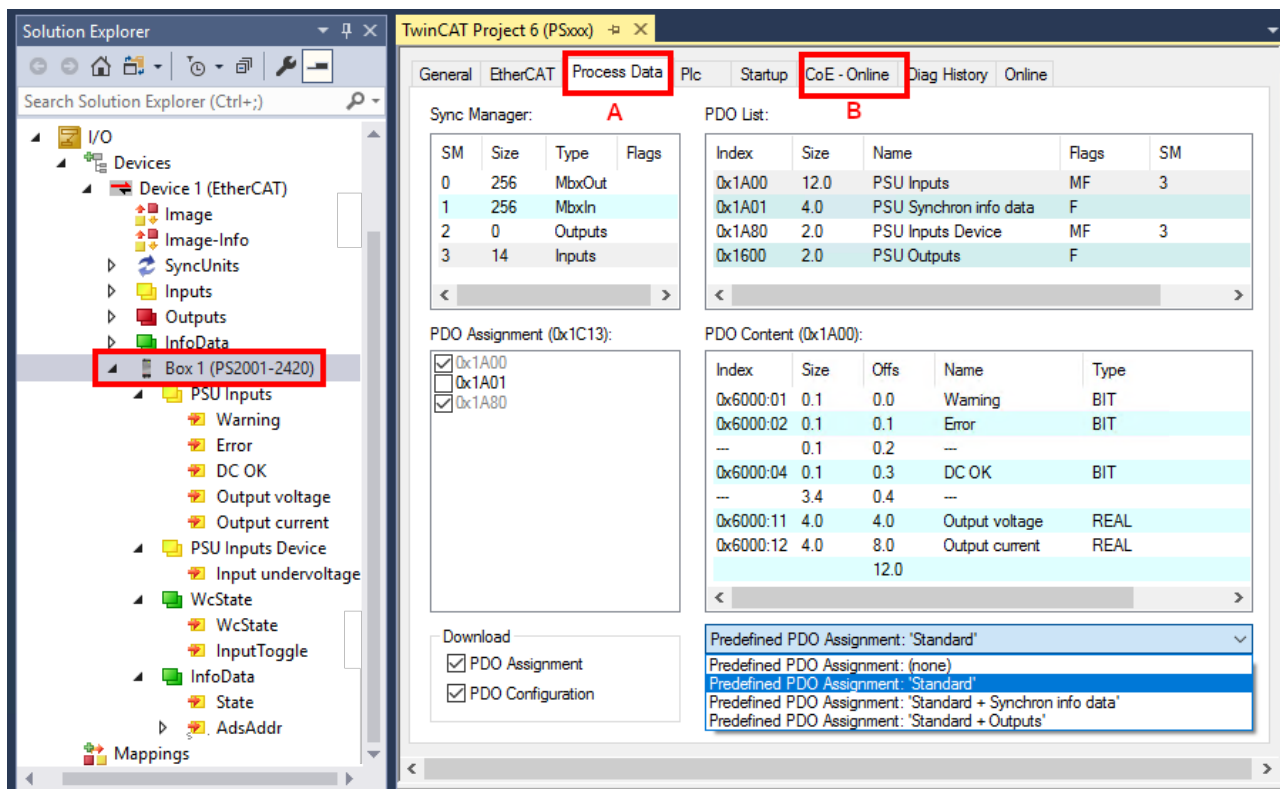
Abb. 133: Parametrierung am Beispiel PS2001-2420-1001
