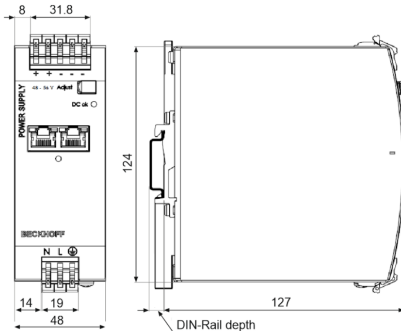
Abb. 16: Vorder-/Seitenansicht PS2001-4810-1001
