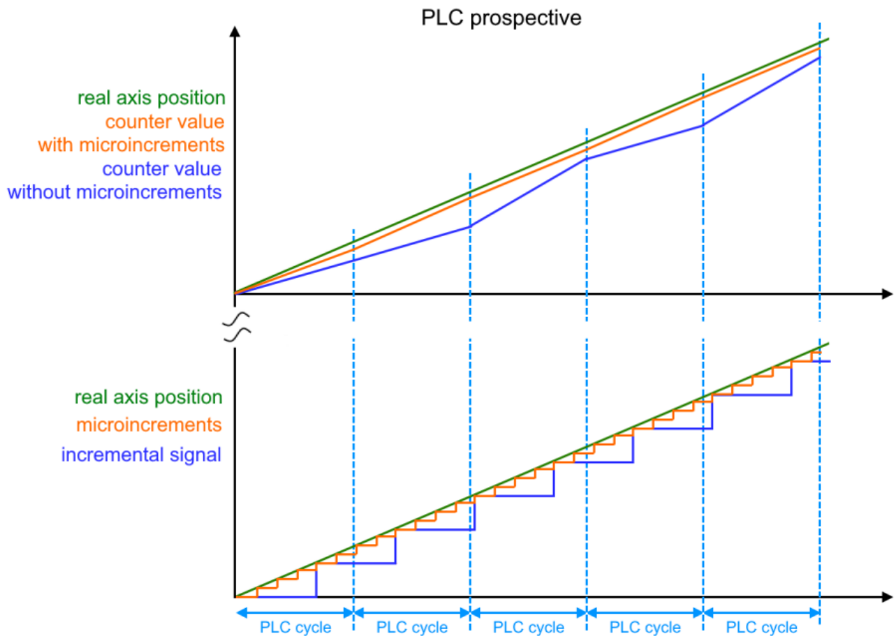
Abb. 169: Funktionsprinzip Mikroinkremente
