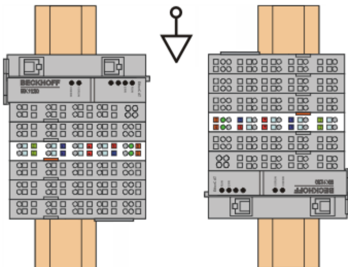
Abb. 26: Weitere Einbautagen, Beispiel 1
