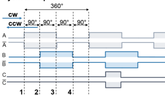
Abb. 8: Inkremental-Signale
