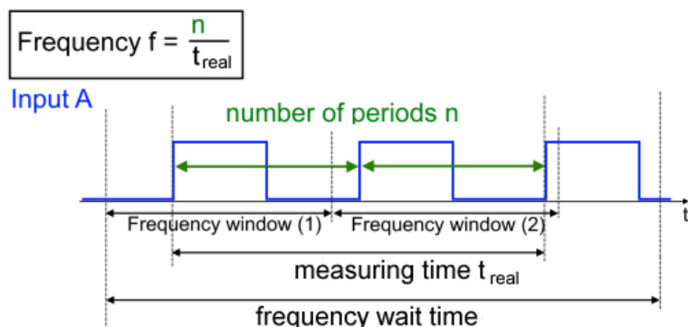
Abb. 165: Frequenzmessung außerhalb des Frequenzfensters mit Wartezeit
