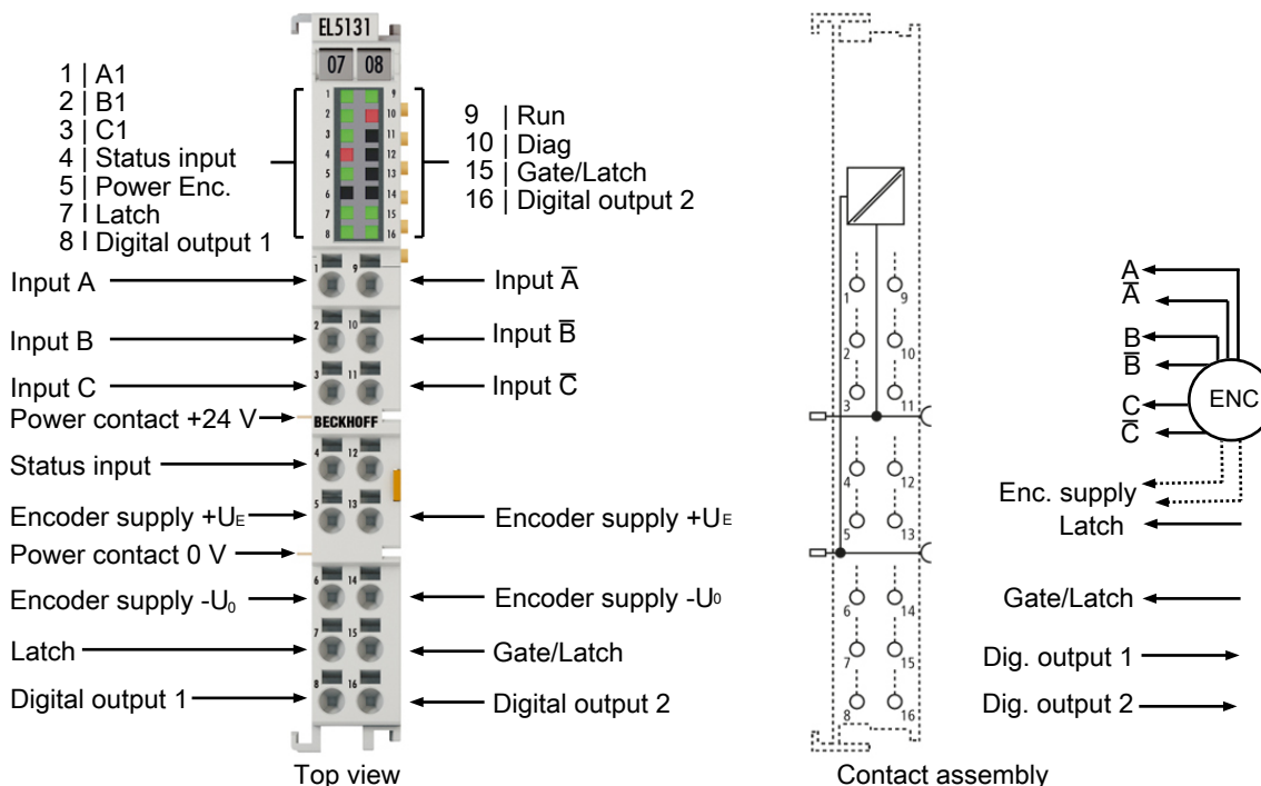
Abb. 4: EL5131
