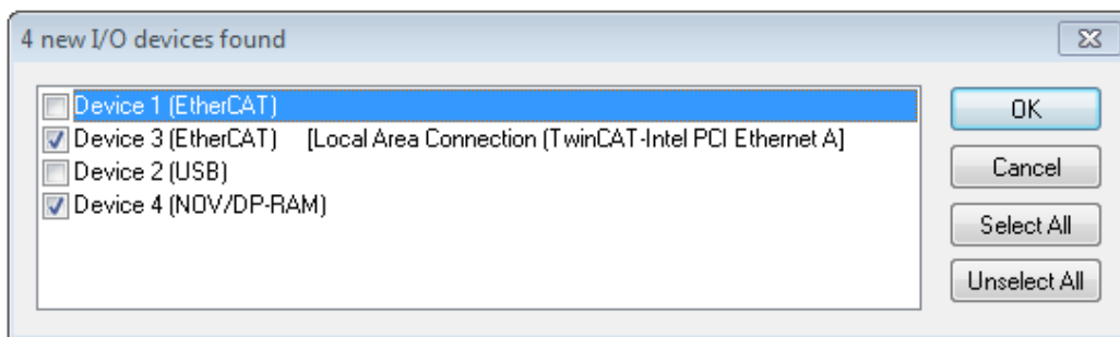
附图 120: 检测到的以太网设备
