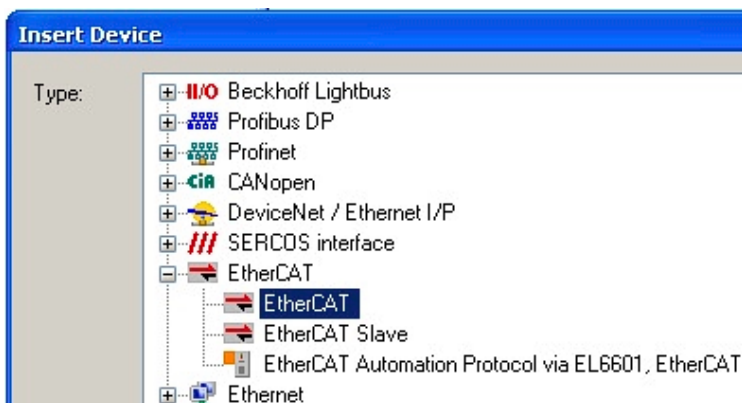
附图 108: 选择 EtherCAT 连接 (TwinCAT 2.11, TwinCAT 3)
