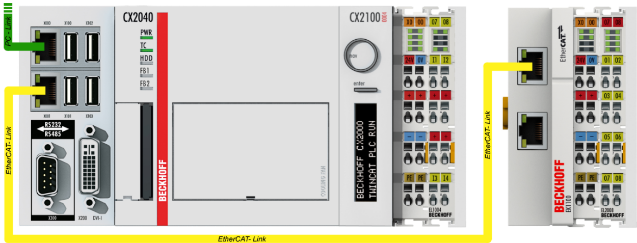
附图 49：控制配置，带嵌入式控制器、输入（EL1004）和输出（EL2008）
