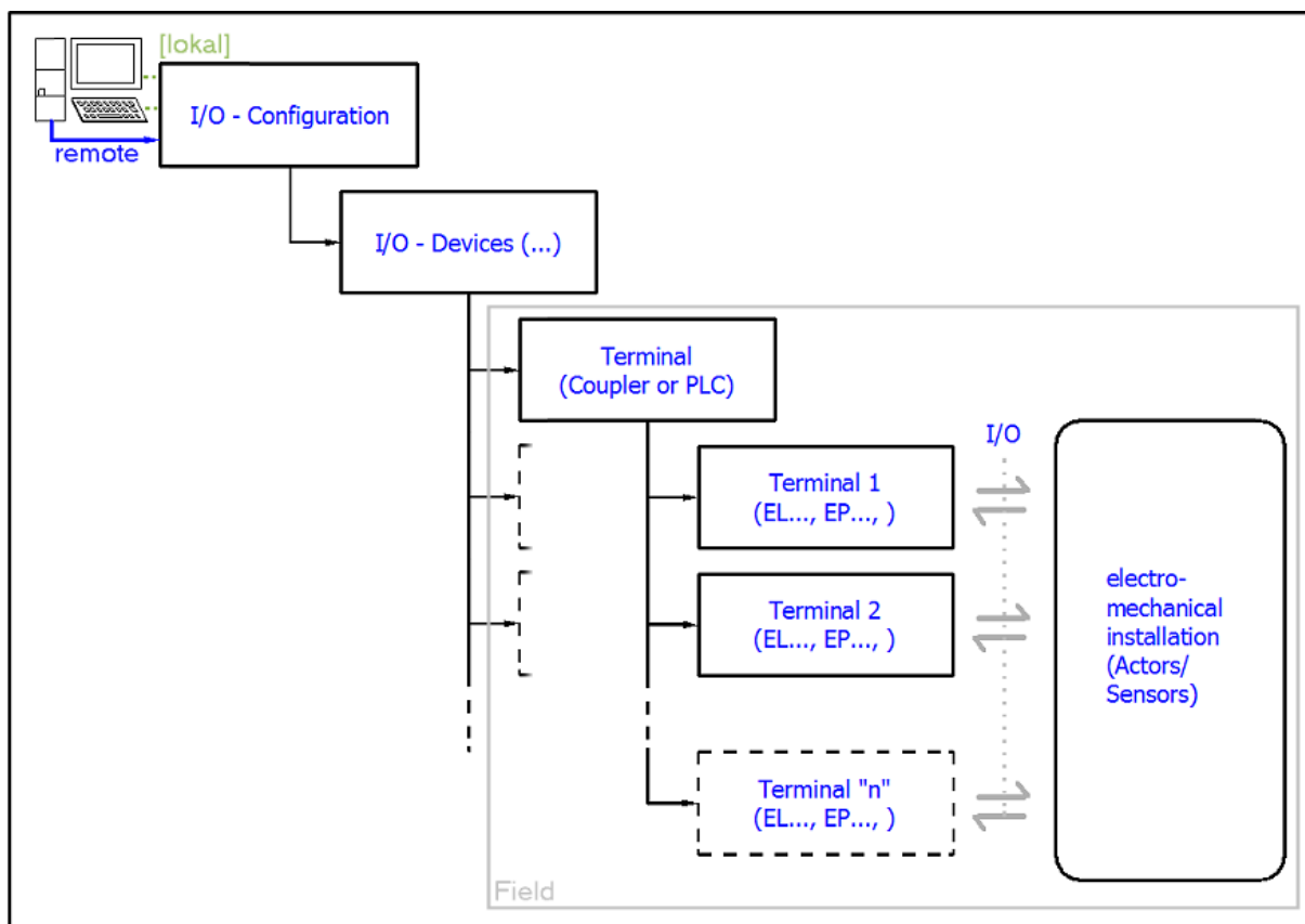
附图 48：用户端（调试）和安装之间的关系
