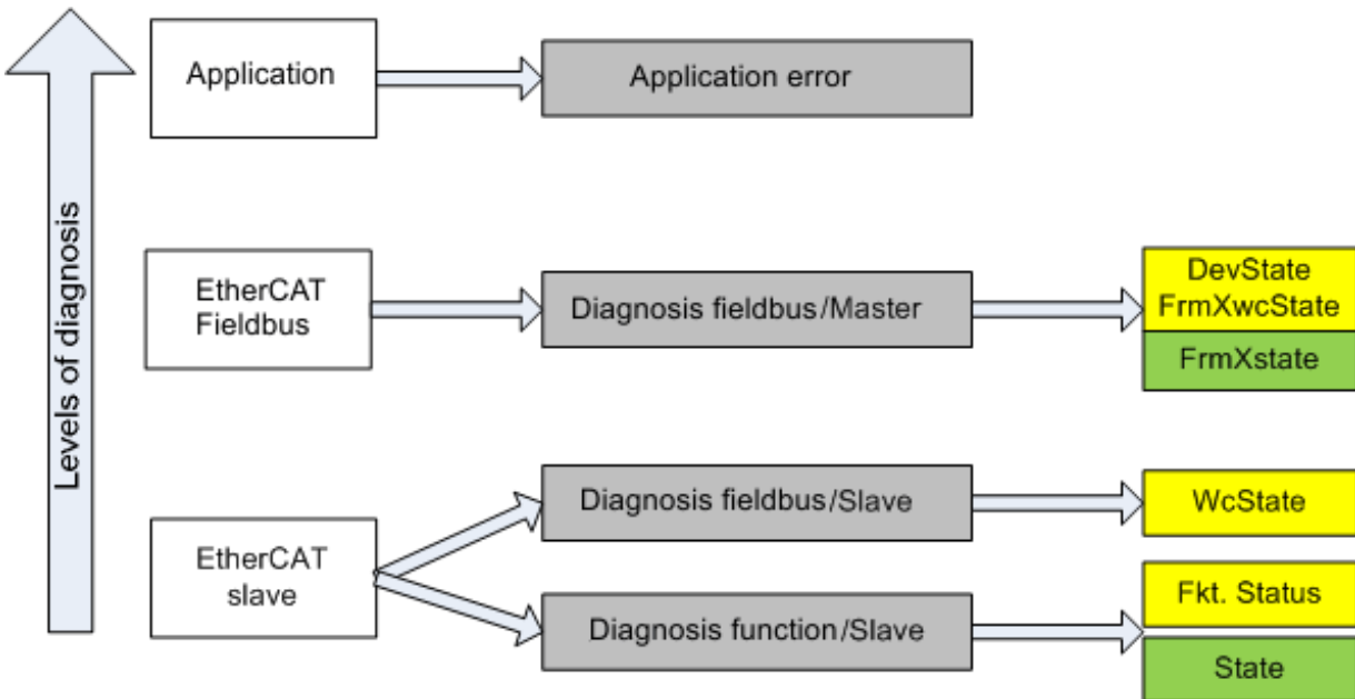
附图 148: 选择 EtherCAT 从站的诊断信息
