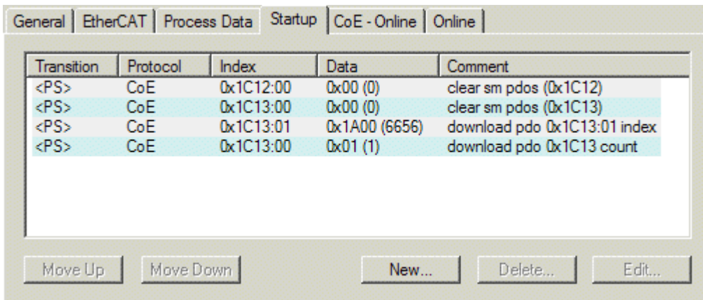
附图 143: “启动”选项卡
