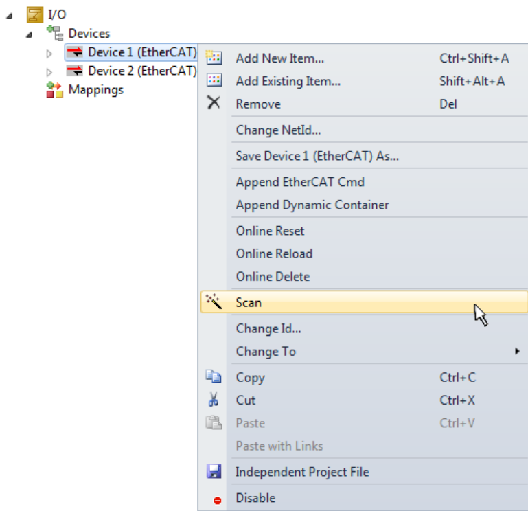
附图 75: 读取连接到设备的单个端子模块
