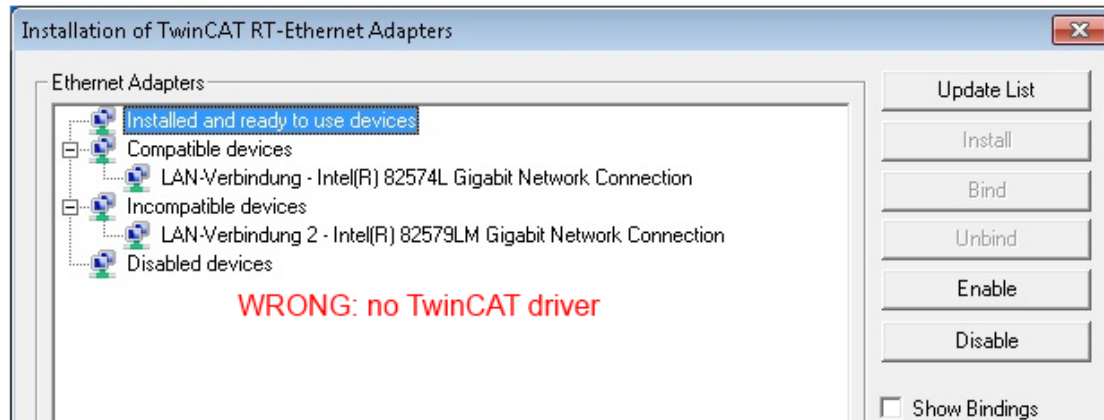
附图 97: 以太网端口的驱动设置不正确
