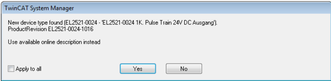
附图 100: 在线描述信息窗口 (TwinCAT 2)
