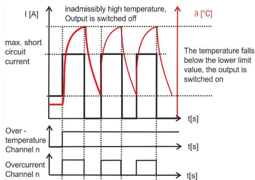
附图 16: 过载情况下的热关机示意图
