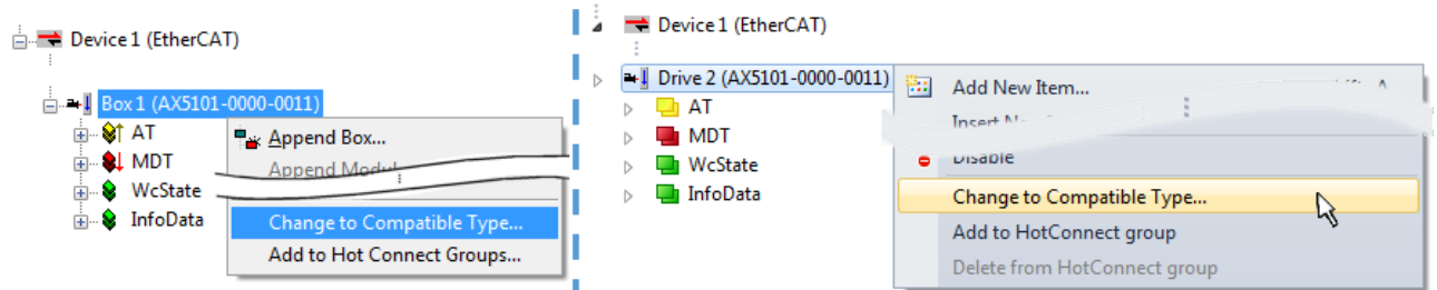
附图 136: 对话框“更改为兼容类型...”（左: TwinCAT 2; 右: TwinCAT 3）
