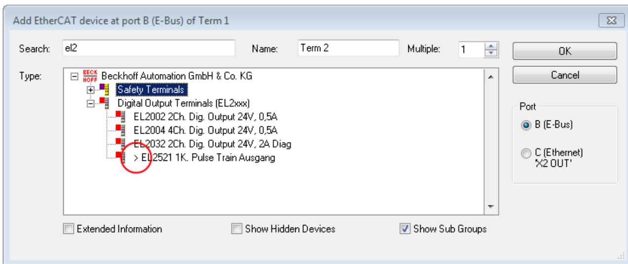
附图 103: 以 EL2521 的在线记录 ESI 为例进行说明
