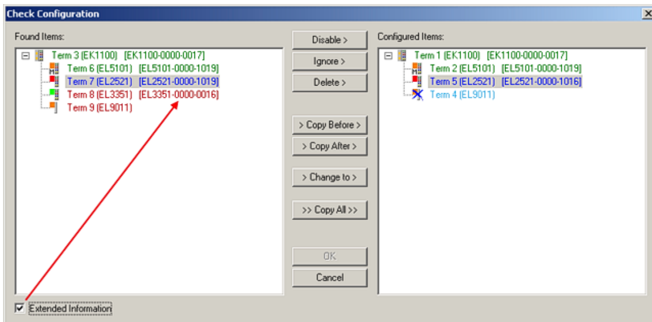
附图 133: 校正对话框
