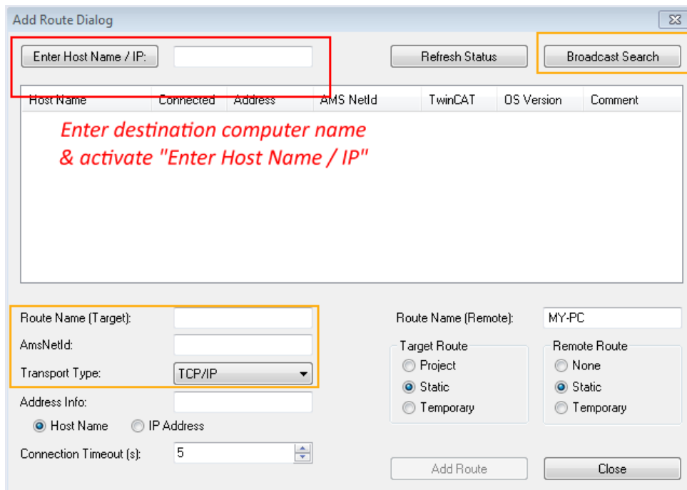
附图 52: 指定通过 TwinCAT 系统管理器访问的 PLC: 选择目标系统
