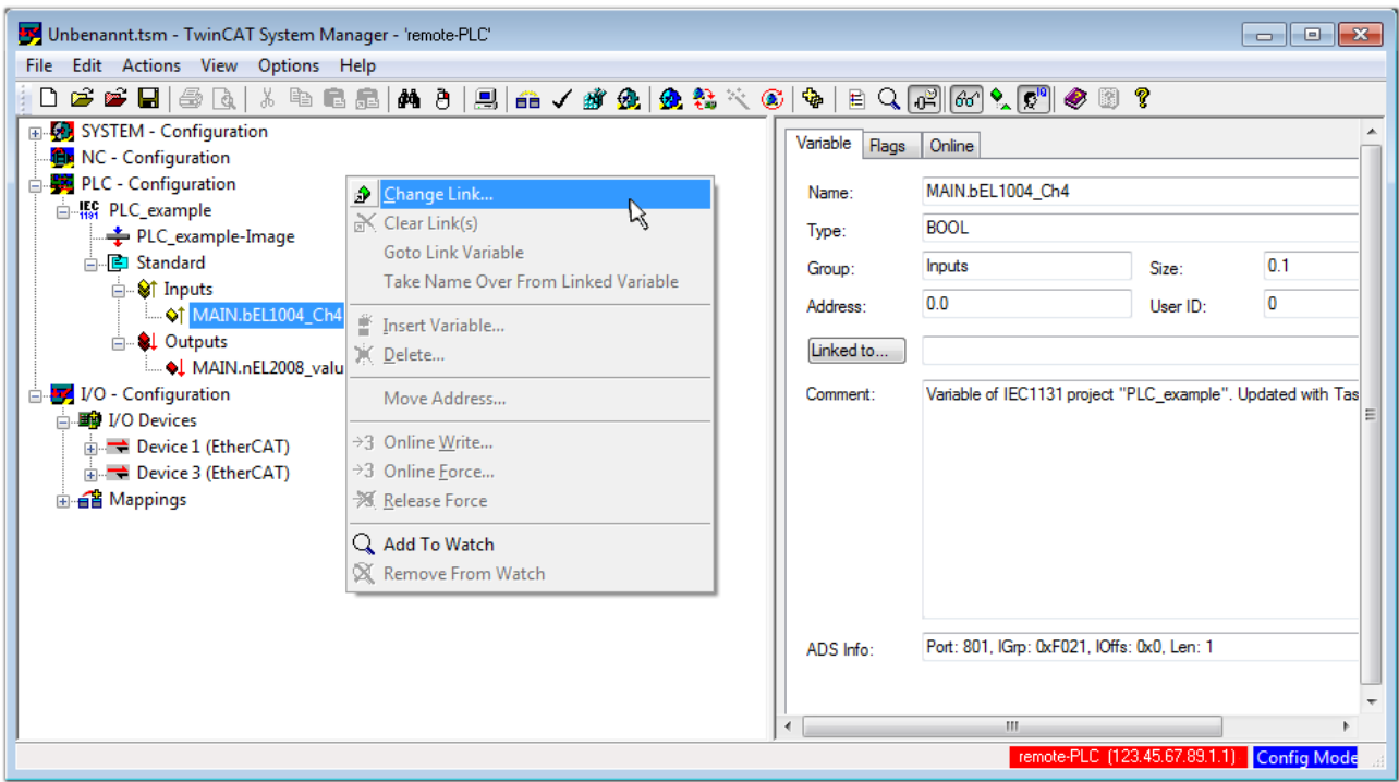
附图 61: 在 PLC 变量和过程对象之间建立链接
