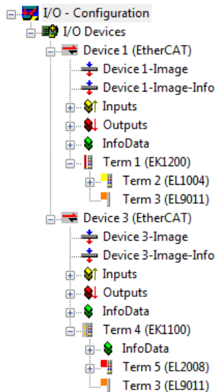
附图 55: TwinCAT 2 系统管理器中的配置映射
