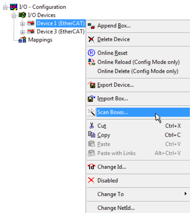
附图 56: 读取连接到设备的单个端子模块
