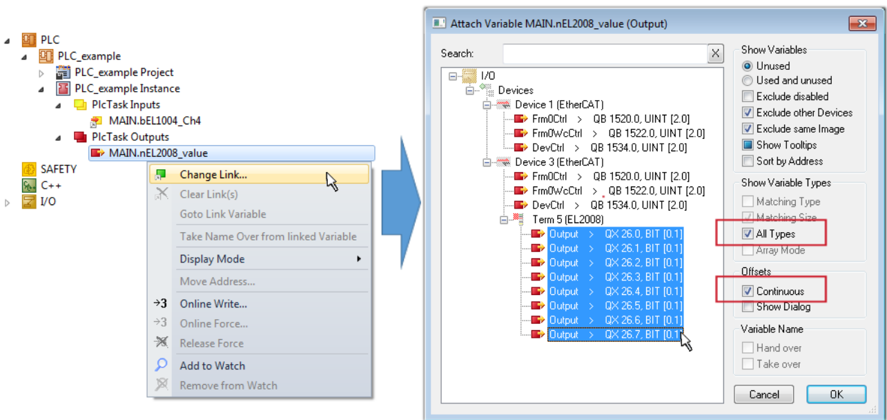
附图 83: 同时选择几个 PDO: 激活“连续”和“所有类型”
