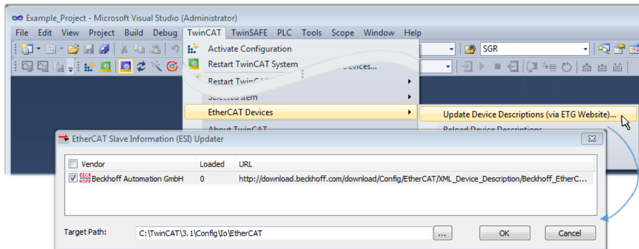
附图 106: 使用 ESI Updater (TwinCAT 3)
