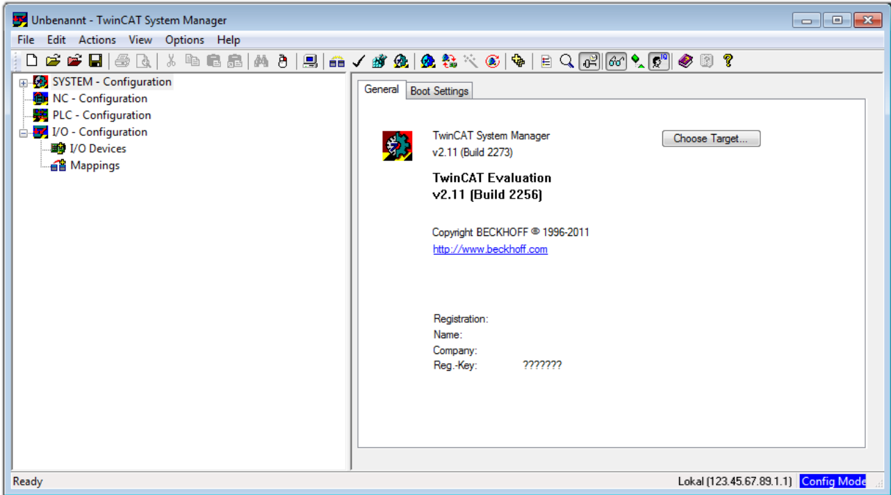
附图 50: 初始 TwinCAT 2 用户界面
