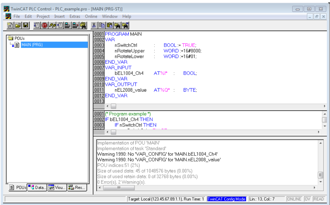
附图 58: 编译过程后带有变量的示例程序（无变量整合）
