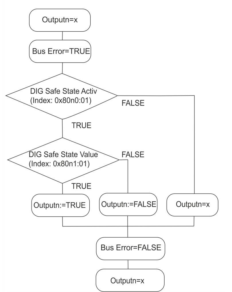
附图 22: 在发生总线错误的情况下改变输出的状态
