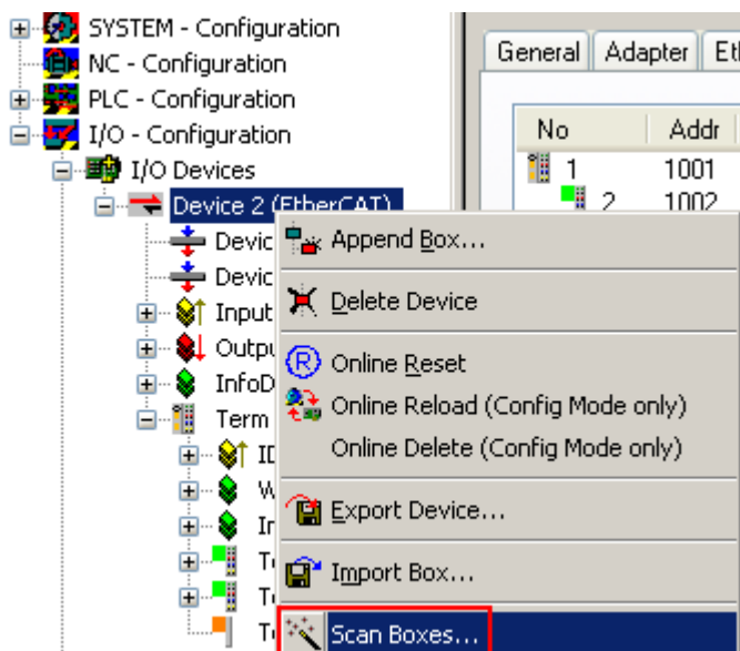
附图 158: 通过右键点击 EtherCAT 设备来扫描下级字段
