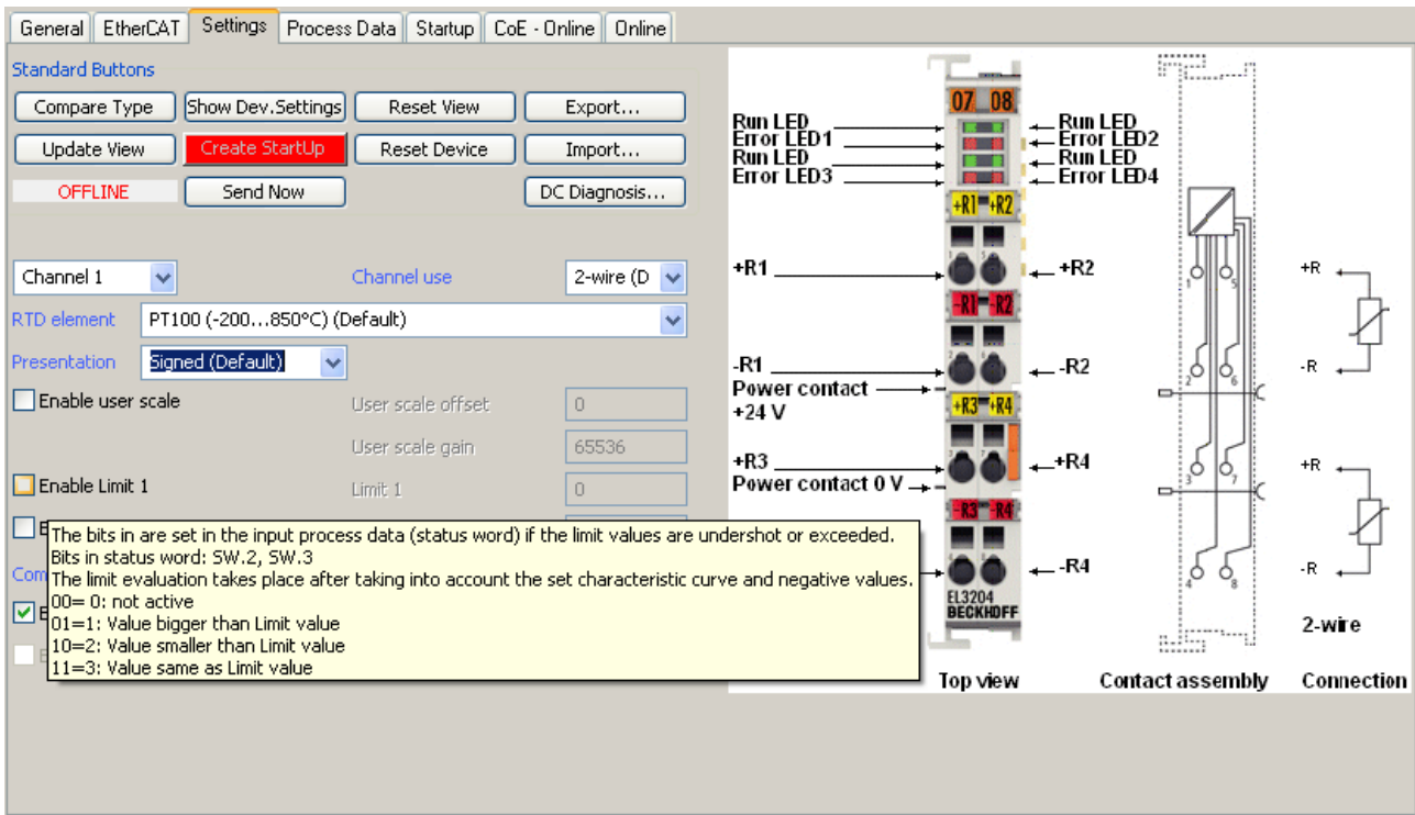
附图 151: EL3204 调试辅助示例
