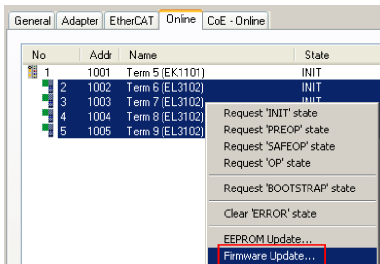
附图 168：多重选择和固件更新
