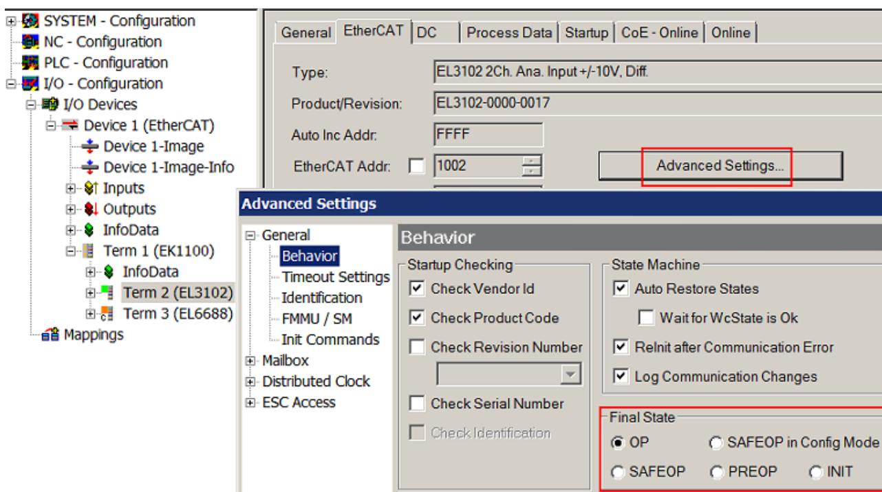
附图 153: 从站的默认目标状态
