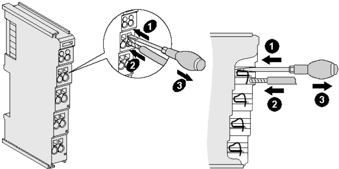
附图 43：在一个接线点上连接电缆
