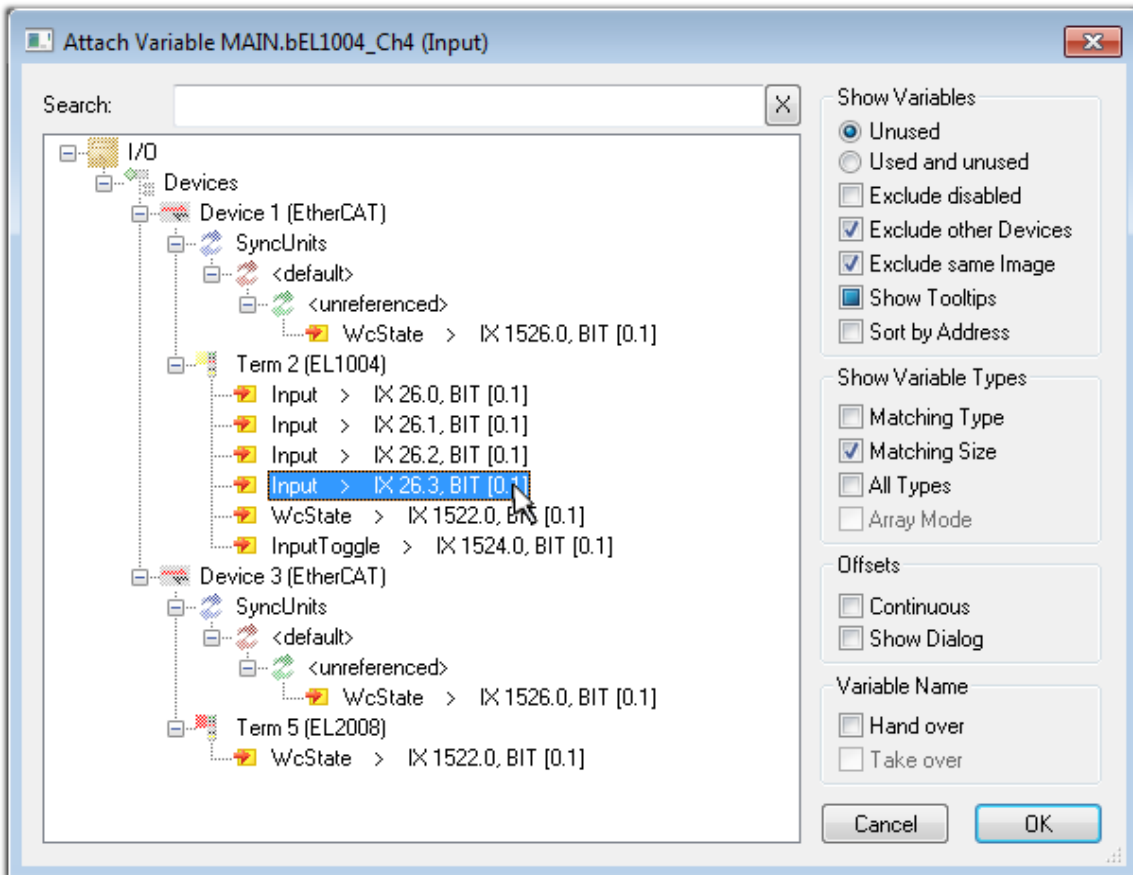
附图 82: 选择 BOOL 类型的 PDO
