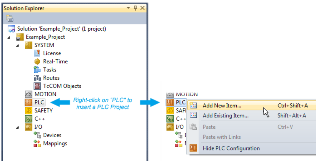
附图 76: 在“PLC”中添加编程环境
