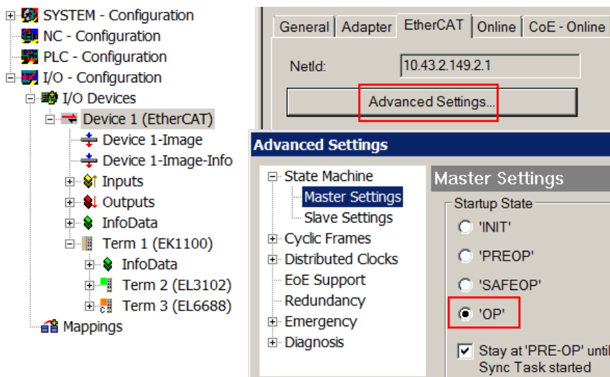
附图 152: 系统管理器的默认行为
