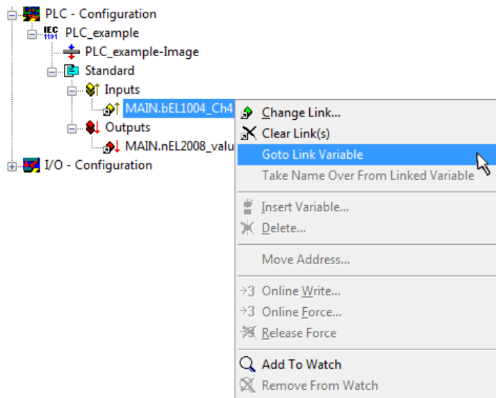
附图 64: 以“MAIN.bEL1004_Ch4”为例，应用“转到链接变量”
