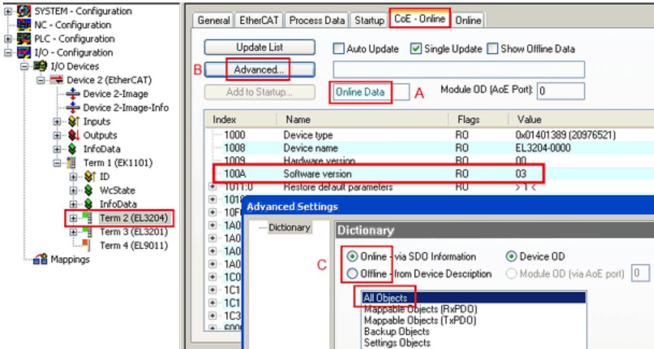
附图 163: EL3204 固件版本的显示
