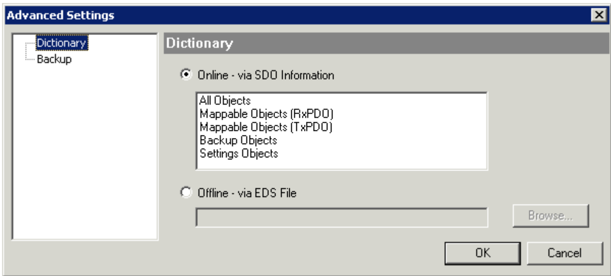
附图 145: “高级设置”对话框
