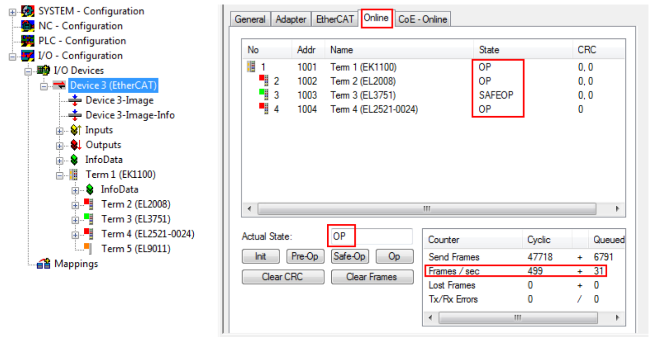
附图 130: 在线显示示例
