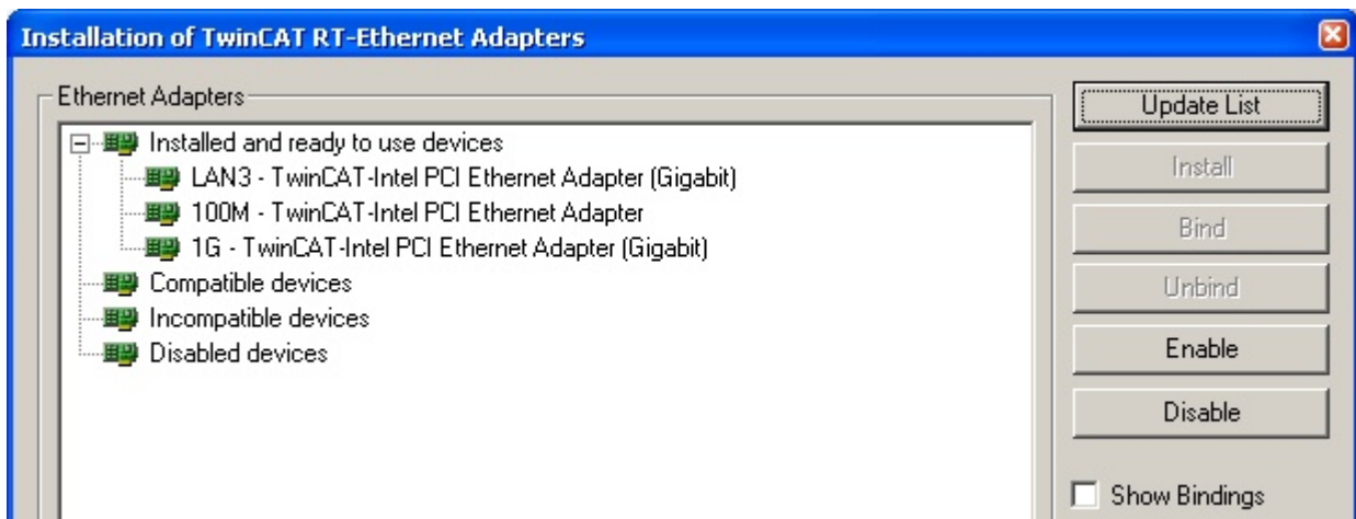
附图 93: 网络接口概述
