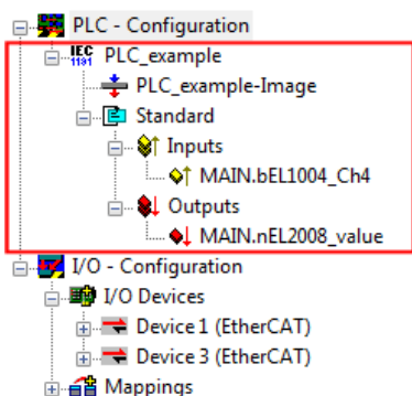
附图 60: 集成在系统管理器 PLC 配置中的 PLC 项目
