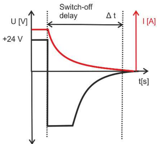
附图 17: 电感负载的关闭
