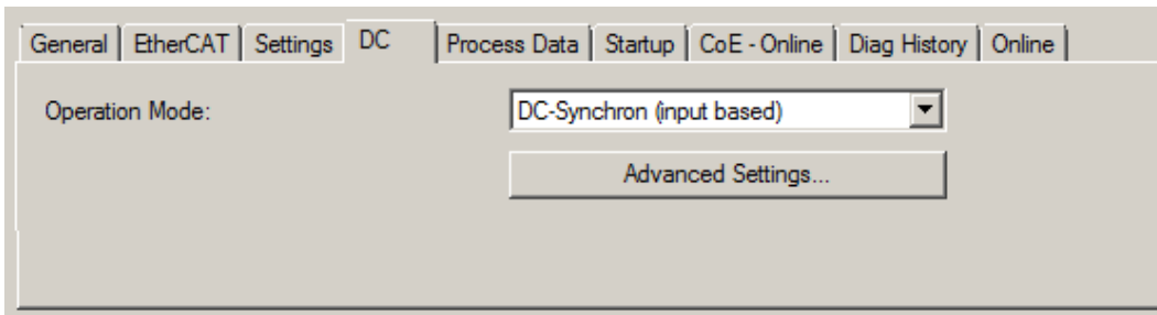
附图 147: “DC”选项卡（分布式时钟）
