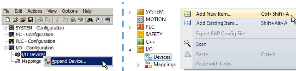
附图 107: 添加 EtherCAT 设备 (左: TwinCAT 2; 右: TwinCAT 3)
