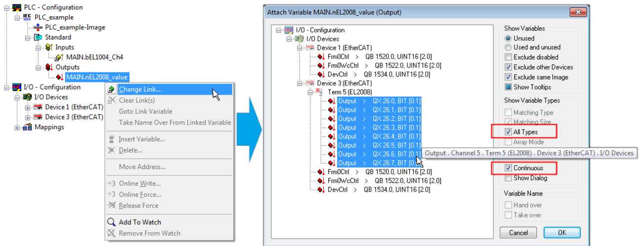
附图 63: 同时选择几个 PDO: 激活“连续”和“所有类型”
