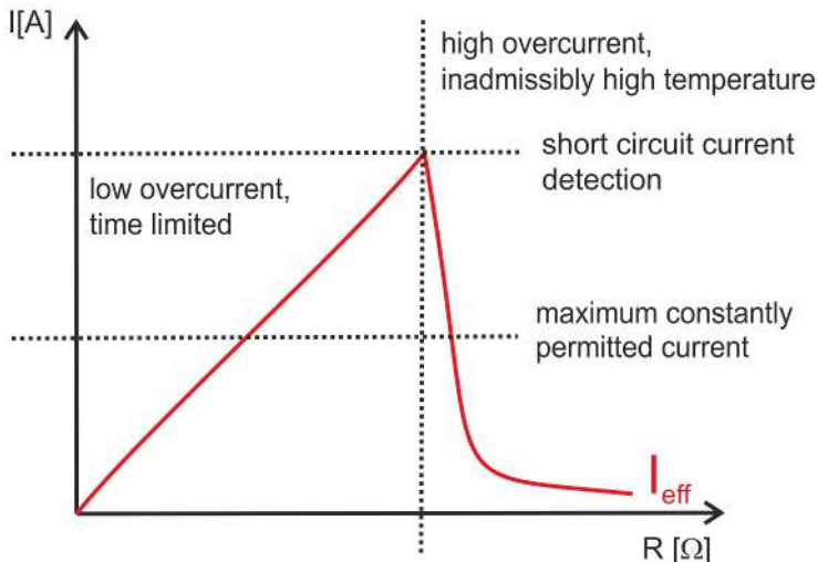
附图 15: 过载电流限制
