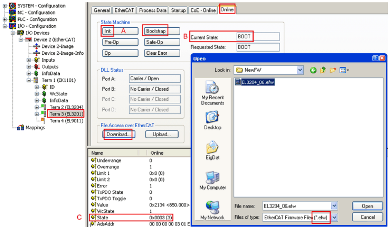
附图 164: 固件更新
