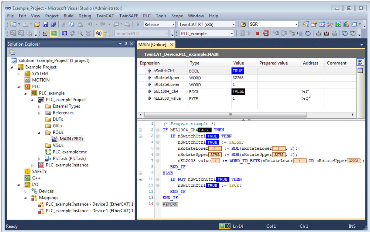
附图 89: TwinCAT 3 开发环境 (VS shell)：程序启动后登录
