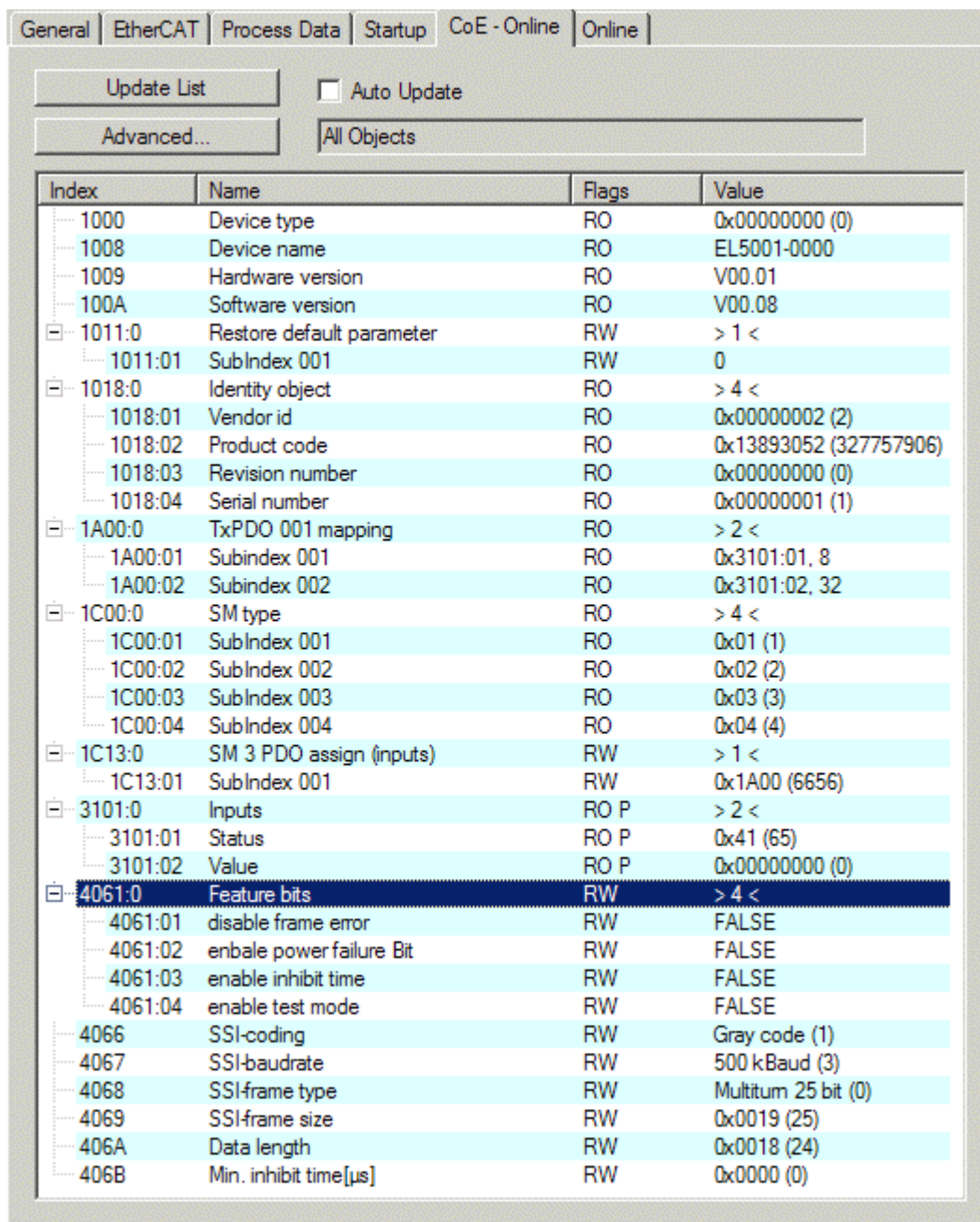
附图 144: “CoE - Online” 选项卡
